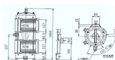
第二種二重式舷灯 NBGS-121
