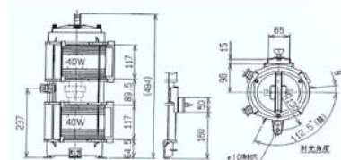
第一種舷灯 二重式NAGS-221
