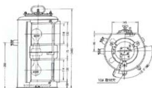
第二種二重式日船式第32号 舷灯
