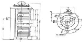
第一種舷灯 二重式日船式C22
