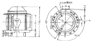
第二種日船式51号 舷灯
